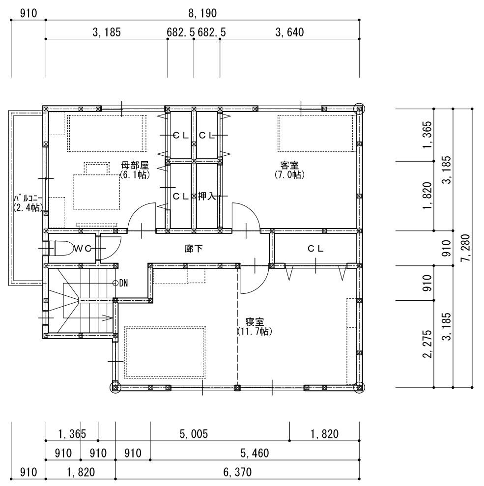
2階平面図
